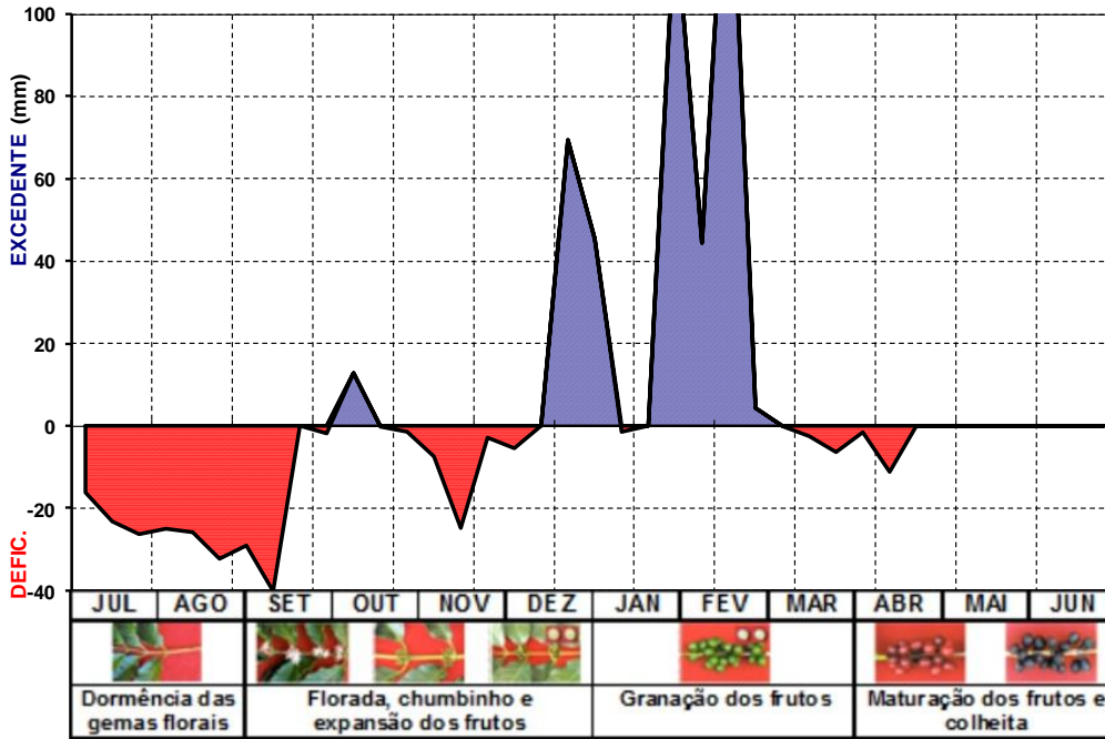
Figura 5 - Balanço hídrico sequencial (Thorntthwaite e Mather, 1955, CAD=100mm) para o ano de 2010/11
