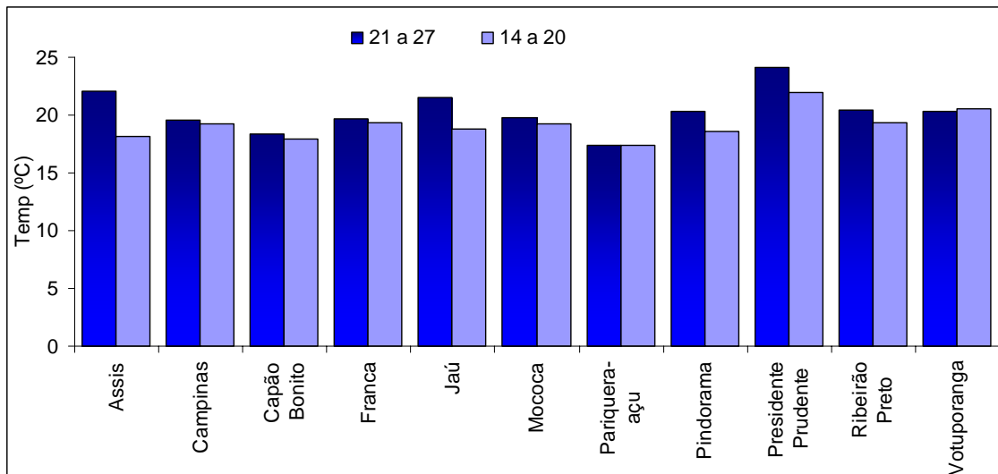
Figura 2 – Temperatura mínima, média do período de 21 a 27/02 comparadas com o período anterior, 14 a 20/02, para localidades do estado de São Paulo.
