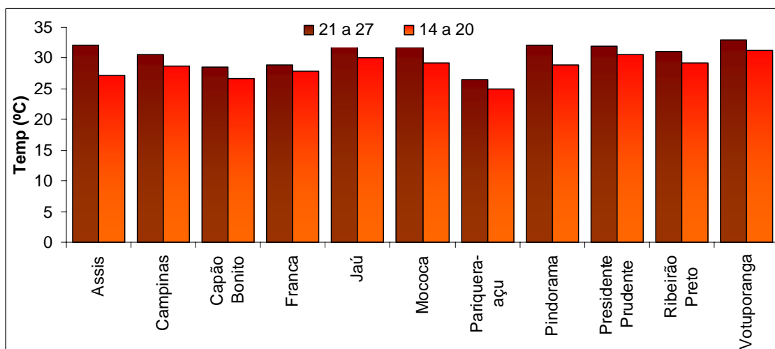
Figura 1 – Temperatura máxima, média do período de 21 a 27/02 comparadas com o período anterior, 14 a 20/02, para localidades do estado de São Paulo.
