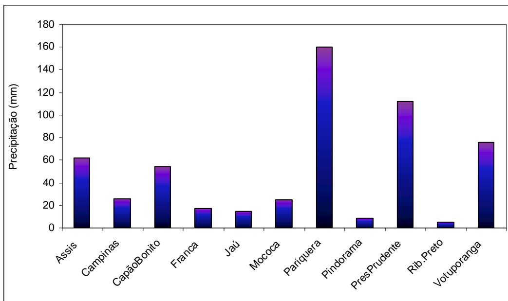
Figura 3 – Volume total de precipitação acumulada no período analisado (21 a 28/02), para localidades do estado de São Paulo. Fonte: Ciiagro.
